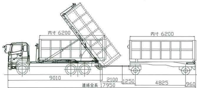
連結図(例) ULTIMA 18S-56
